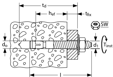
FWA, горячеоцинкованная сталь с клипсой из нержавеющей стали A2
