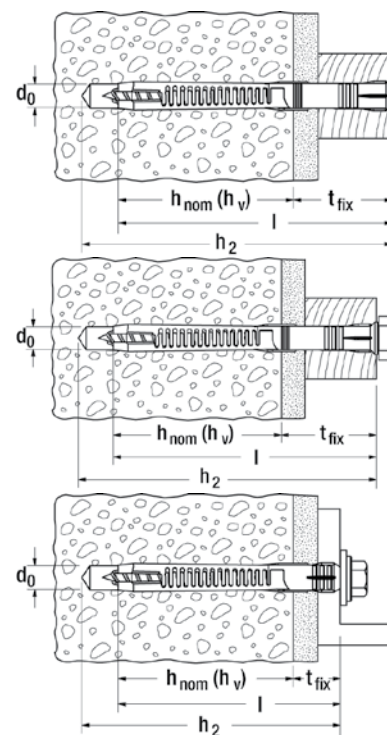
FUR 10 FUS — шуруп с шестигранной головкой и пресс-шайбой
