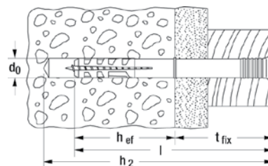
Гвоздевой дюбель N-S A2 с гвоздем из нержавеющей стали A2, предварительно собран
