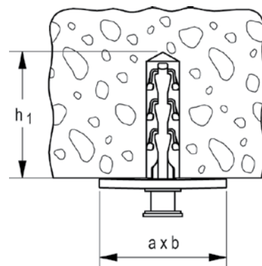
Монтажный прижимной фиксатор-дюбель SF plus MS
