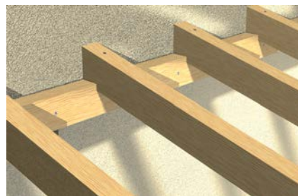
Деревянные конструкции
